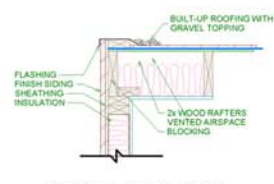
CURBED ROOF EDGE
